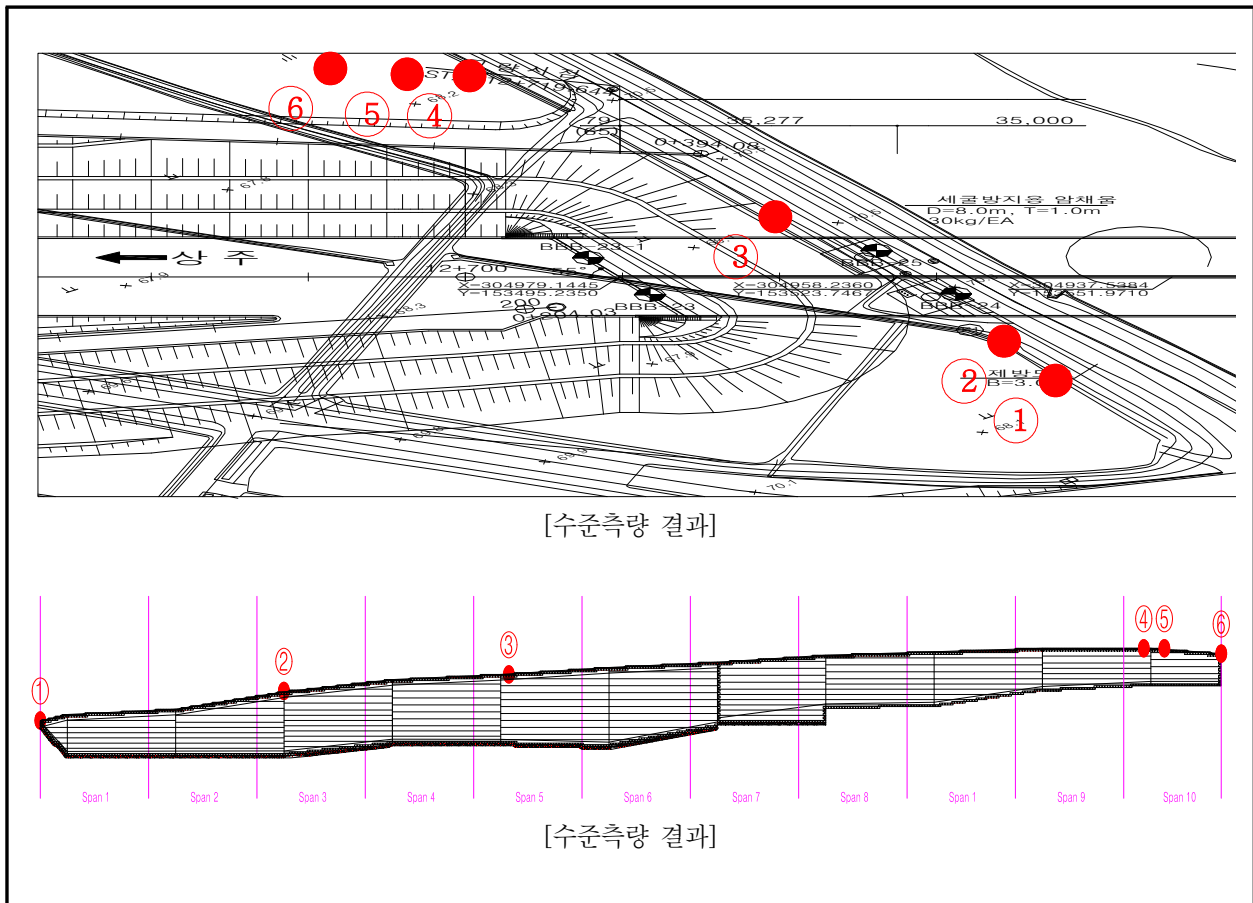
【그림 3.3.5】 선형 및 수준측량 결과
